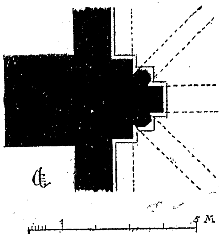
Fig. 16. — Plan du sommet des voûtes de la nef (Sainte-Trinité, à Laval).
