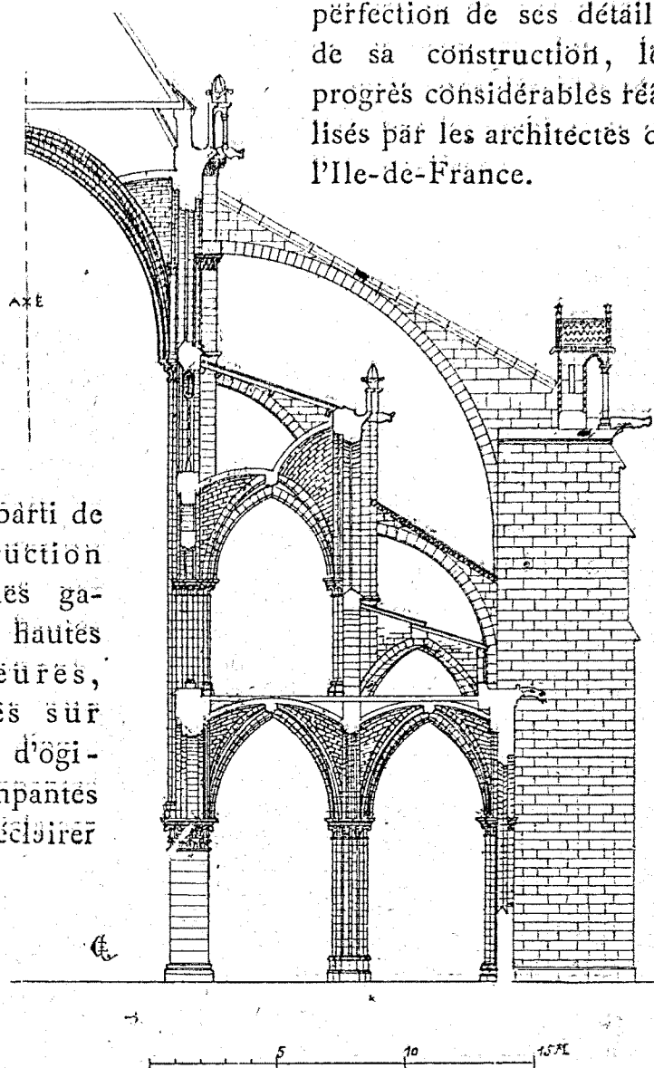
Fig. 37. — Notre-Dame de Paris. — Coupe de la nef.
