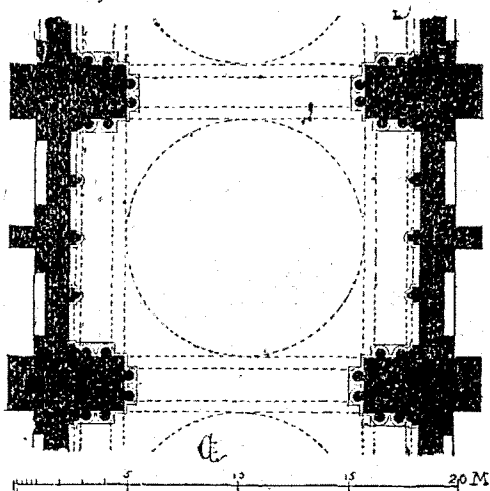
Fig. 4. — Plan d'une des coupes d'Angoulême ou de Fontevrault.
