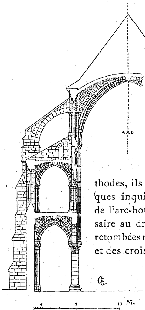
Fig. 36. — Église de Laon. Coupe sur la nef.
