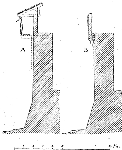
Fig. 170 bis. Hourds en bois et en pierre.
