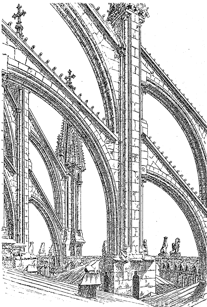
Fig. 46. — Cathédrale de Reims — Arcs-boutants du chœur.
