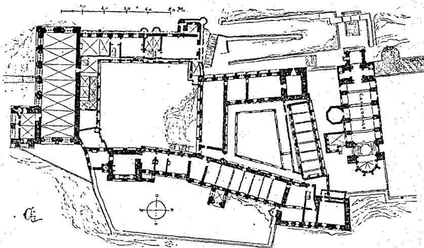
Fig. 235. — Palais des Papes à Avignon. — Plan.
