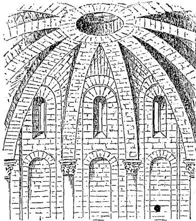
Fig. 28. — Église du Moutier, à Moissac. Voûte de la salle, dite des Capitaines, au-dessus du porche.
