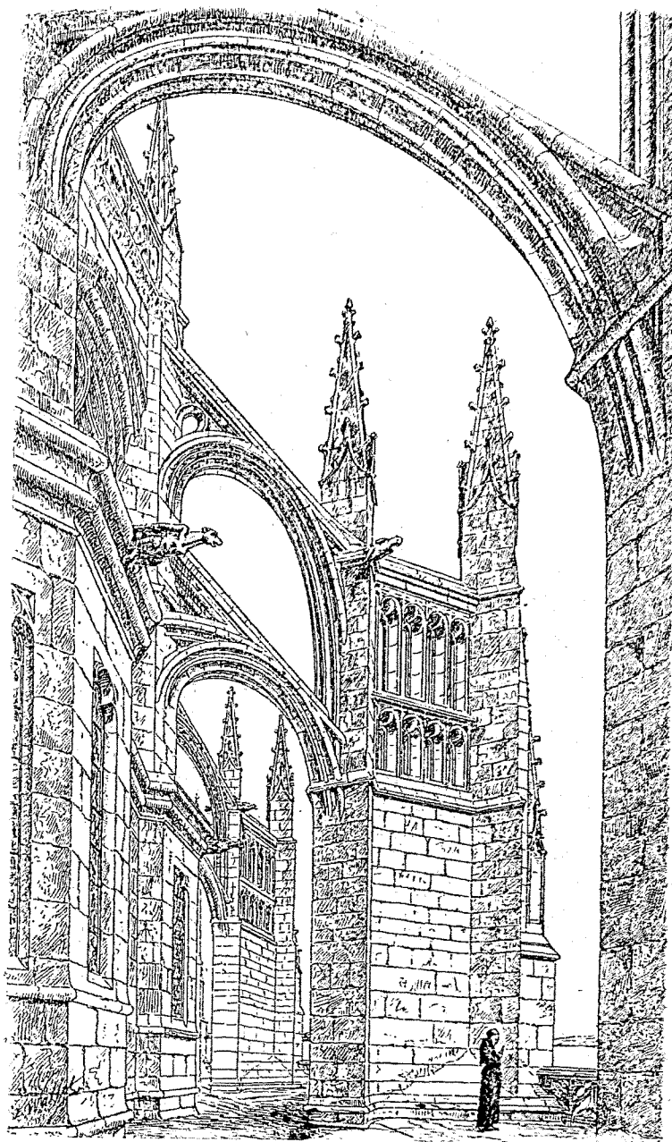
Fig. 75. — Abbaye du Mont-Saint-Michel. Arcs-boutants du chœur (fin du xve siècle). (D'après les dessins d'Ed. Corroyer.)
