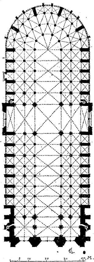
Fig. 37. — Notre-Dame de Paris. Plan.
