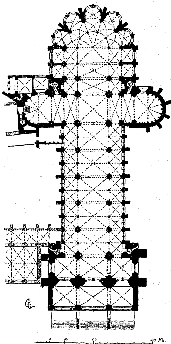
Fig. 25. — Église de Noyon. — Plan.
