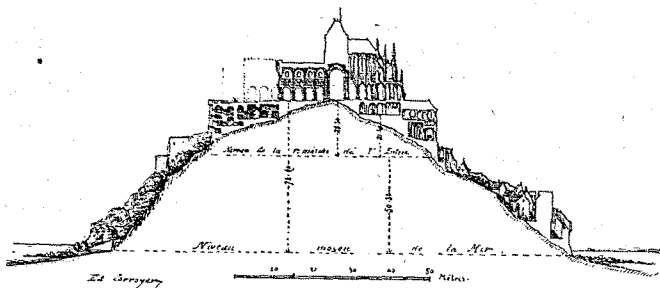
Fig. 154. — Abbaye du Mont-Saint-Michel. — Coupe longitudinale, de l'ouest à l'est.
