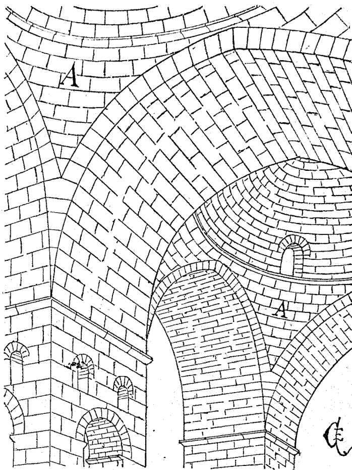
Fig. 2. — Pendentif (en A) d'une des coupôles de l'église abbatiale de Saint-Front.
