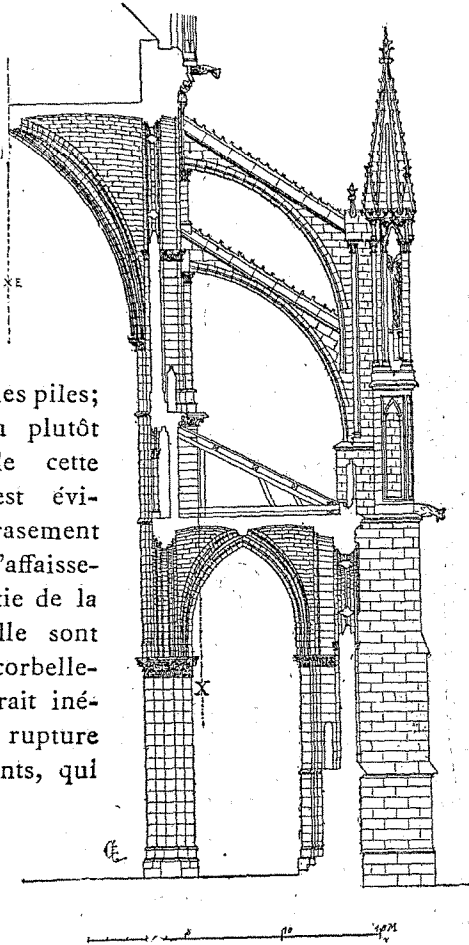
Fig. 45. — Cathédrale de Reims. Coupe sur la nef.
