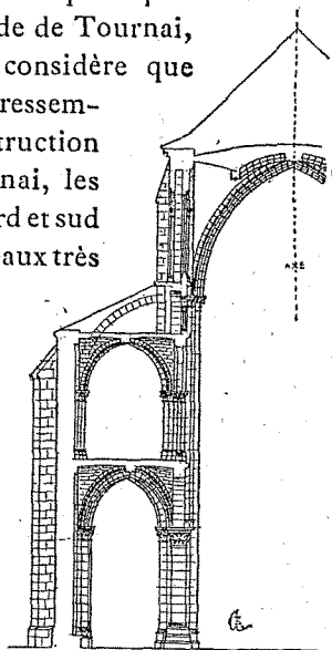
Fig. 26. — Église abbatiale d Noyon. — Coupe transversale.
