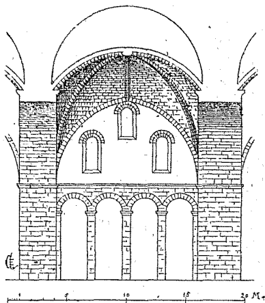
Fig. 6. — Coupe d'une travée de l'église de Saint-Avit-Sénieur.
