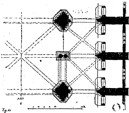
Fig. 40. — Cathédrale de Sens.
