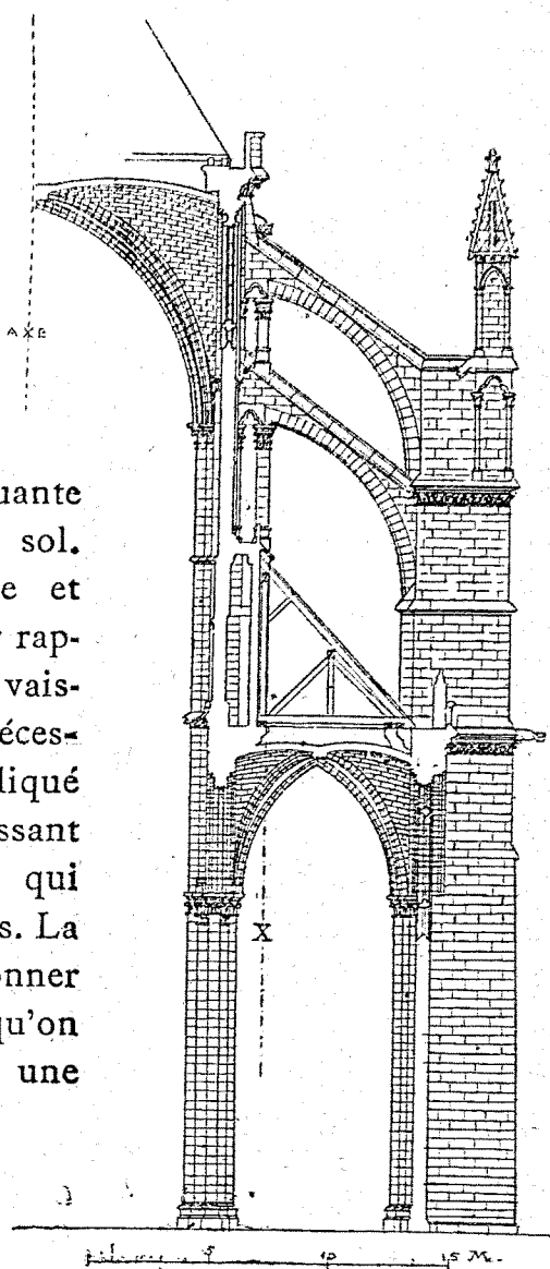
Fig. 48. — Cathédrale d'Amiens. Coupe sur la nef. — Arcs-boutants.
