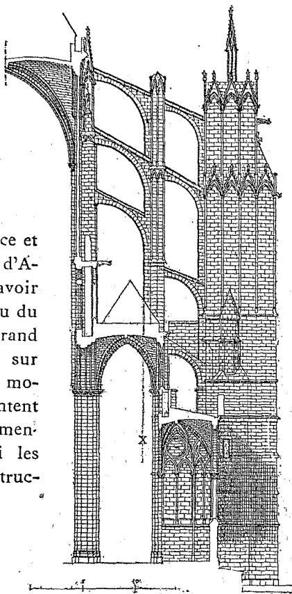
Fig. 51. — Cathédrale de Beauvais. Coupe transversale.
