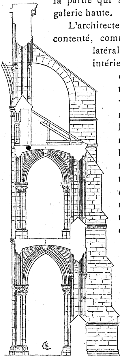
Fig. 30. — Cathédrale de Soissons. Transsept sud. Coupe de l'arc-boutant.
