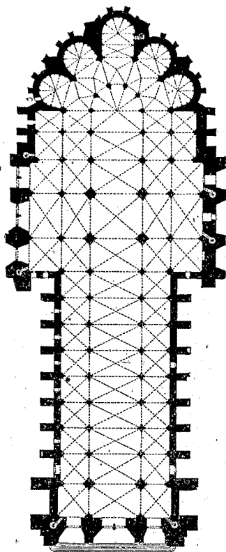
Fig. 77. — Cathédrale de Reims. Plan.
