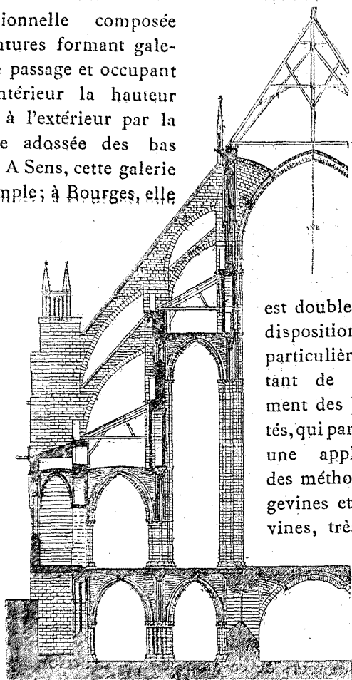
Fig. 43. — Cathédrale de Bourges. — Coupe sur la nef.
