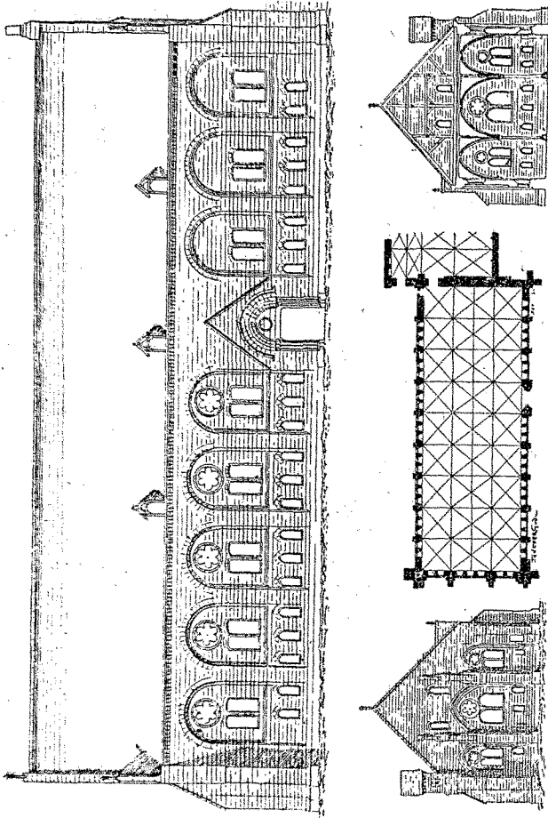
Fig. 203. — Abbaye d'Ourcamps (Oise), — xii e siècle. — Hôpital d'après les relevés d'A. Verdier.
