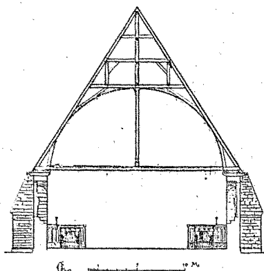
Fig. 207. — Hôpital de Tonnerre. Coupe de la grande salle des malades.
