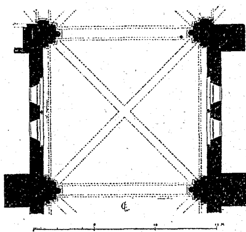
Fig. 9. — Plan d'une travée de l'église d'Angers (Saint-Maurice).
